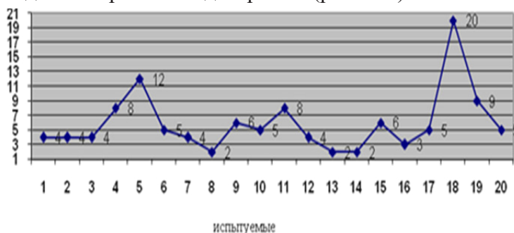
Рис. №1. Количественные показатели уровня переключаемости внимания среди (учащиеся 4 классов).
